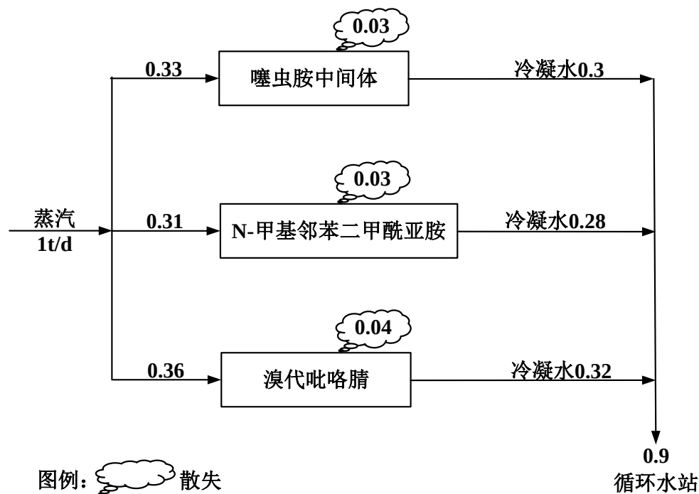
图 3.3-4 全厂蒸汽/凝水平衡图 单位：t/h
