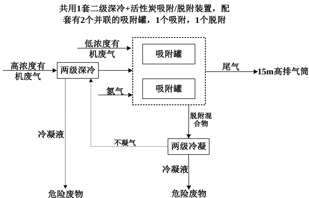
图 3.5-1 两级深冷+活性炭吸附/脱附装置工艺流程图
