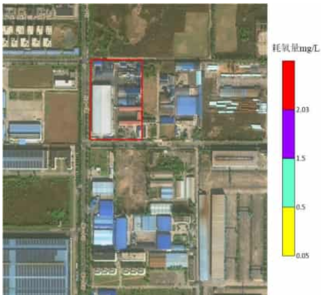
图 5.6-18 7300 天污染晕运移分布图
