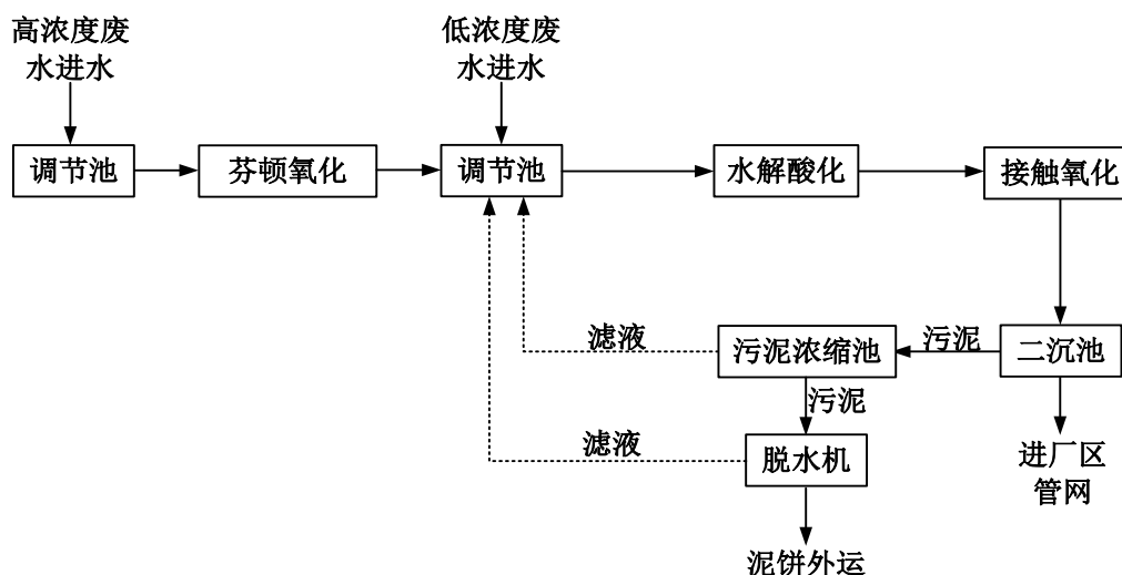
图 7.2-1 厂区污水站废水治理工艺流程图
