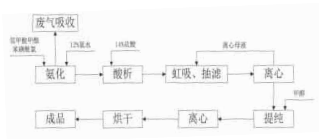
图 3.2-1 邻磺苯甲酰亚胺生产工艺流程及产污环节示意图
