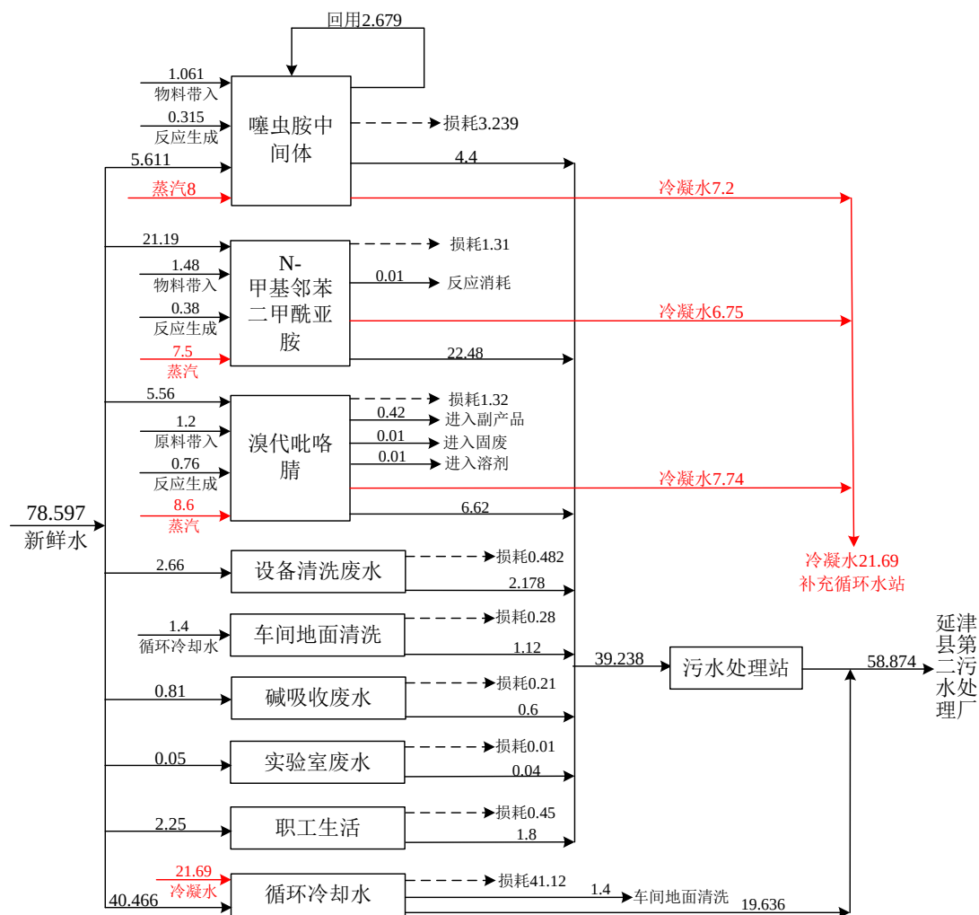
图 3.3-2 全厂水平衡图 单位: \text{m}^3/\text{d}
