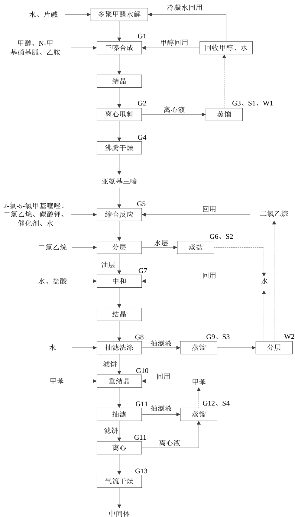
图 3.2-2 噻虫胺中间体生产工艺流程及产污环节示意图
