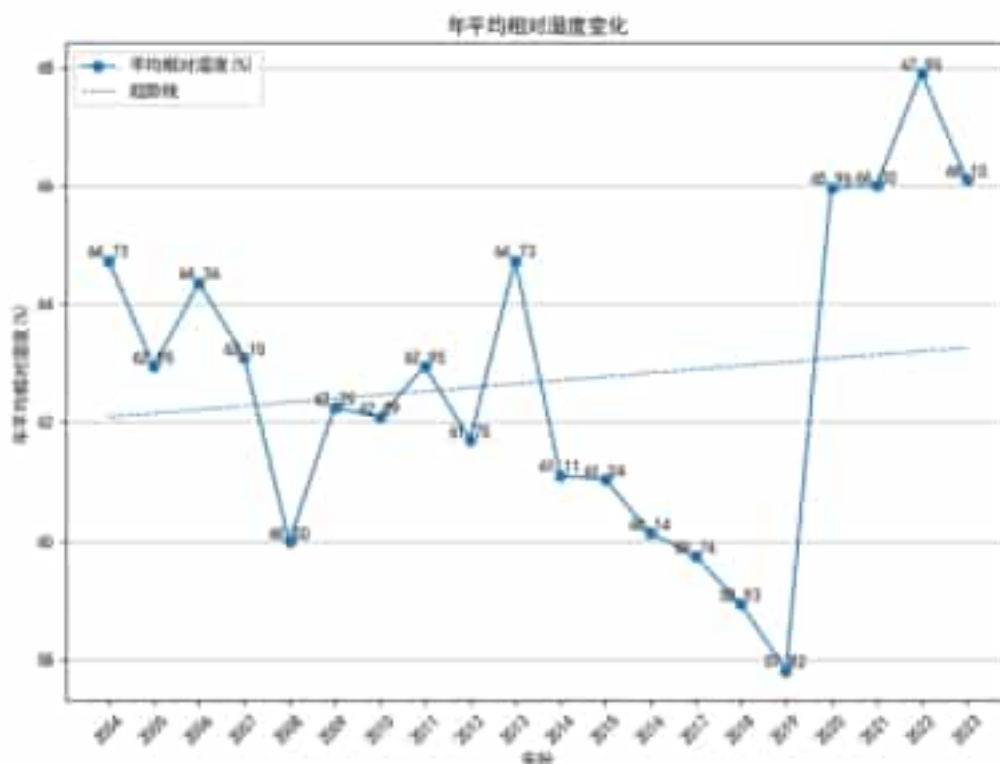
图 5.2-9 新乡（2004-2023）年平均相对湿度（纵轴为百分比，虚线为趋势线）
