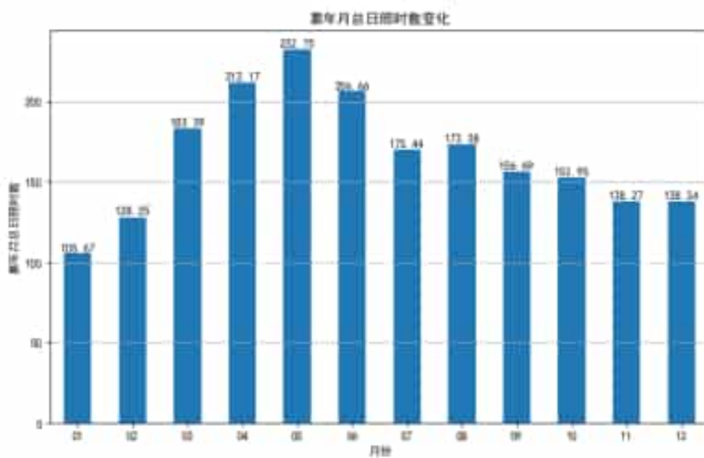
图 5.2-10 新乡月日照时数（单位：小时）
