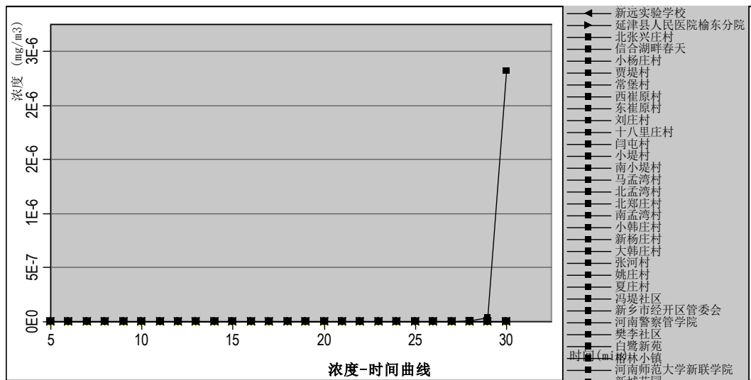
图 6.2-25 最不利气象敏感点三氯化磷浓度-时间曲线
