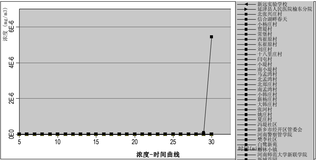
图 6.2-48 最常见气象敏感点 CO 浓度-时间曲线
