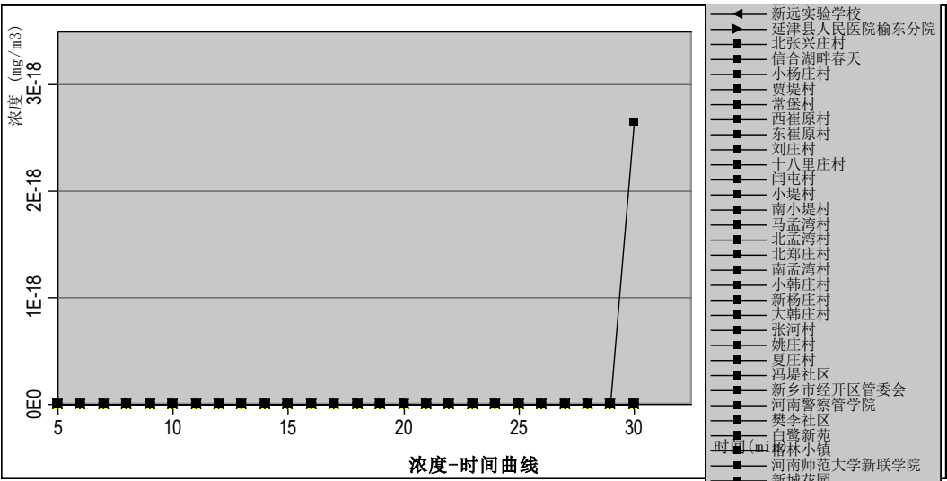
图 6.2-21 最不利气象敏感点 DMF 浓度-时间曲线
