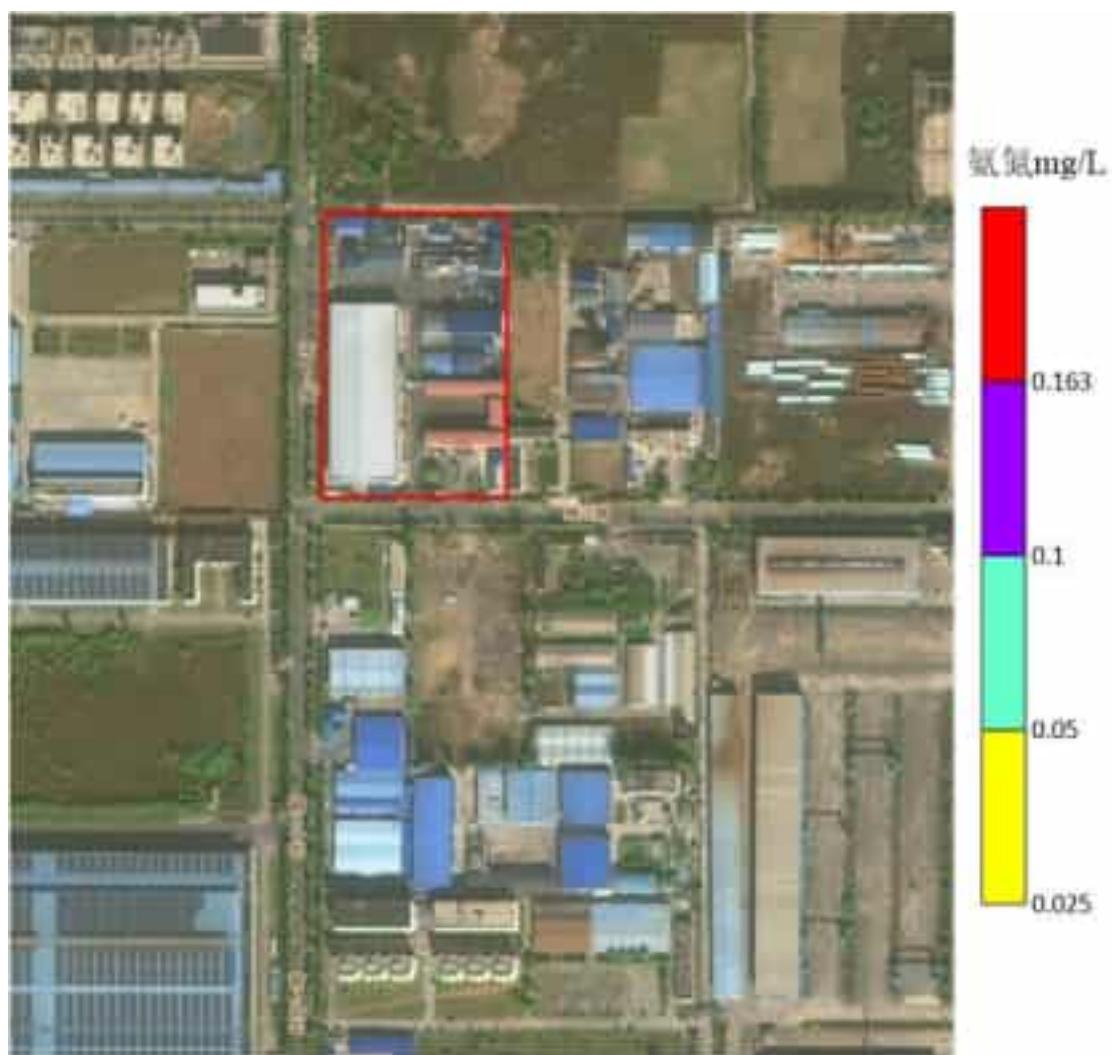
图 5.6-21 3650 天污染晕运移分布图
