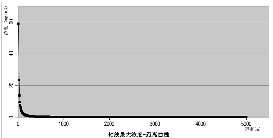
图 6.2-12 最常见气象下风溴化氢最大浓度-距离曲线
