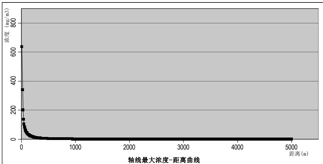
图 6.2-15 最不利气象下风向甲苯最大浓度-距离曲线
