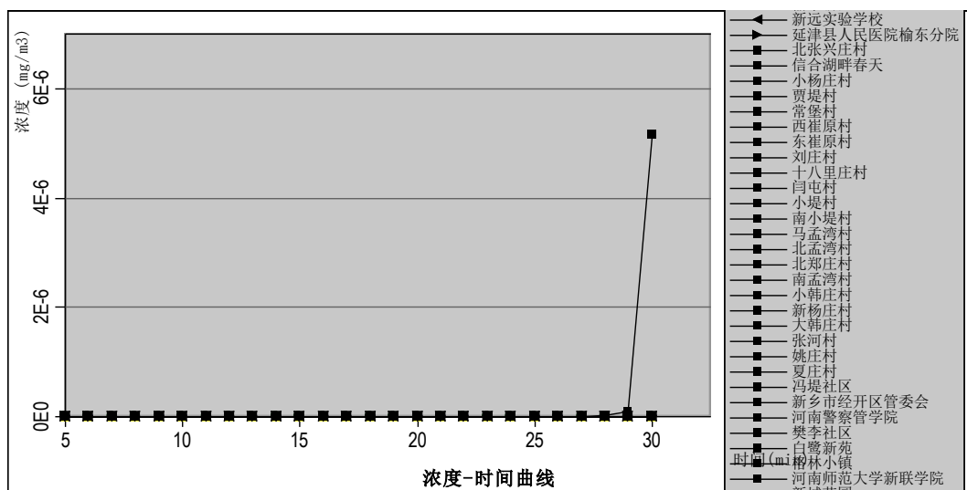
图 6.2-30 最常见气象敏感点氯化氢浓度-时间曲线
