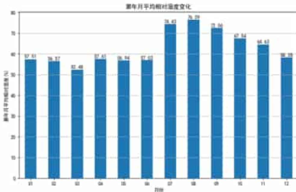
图 5.2-8 新乡月平均相对湿度（纵轴为百分比）
