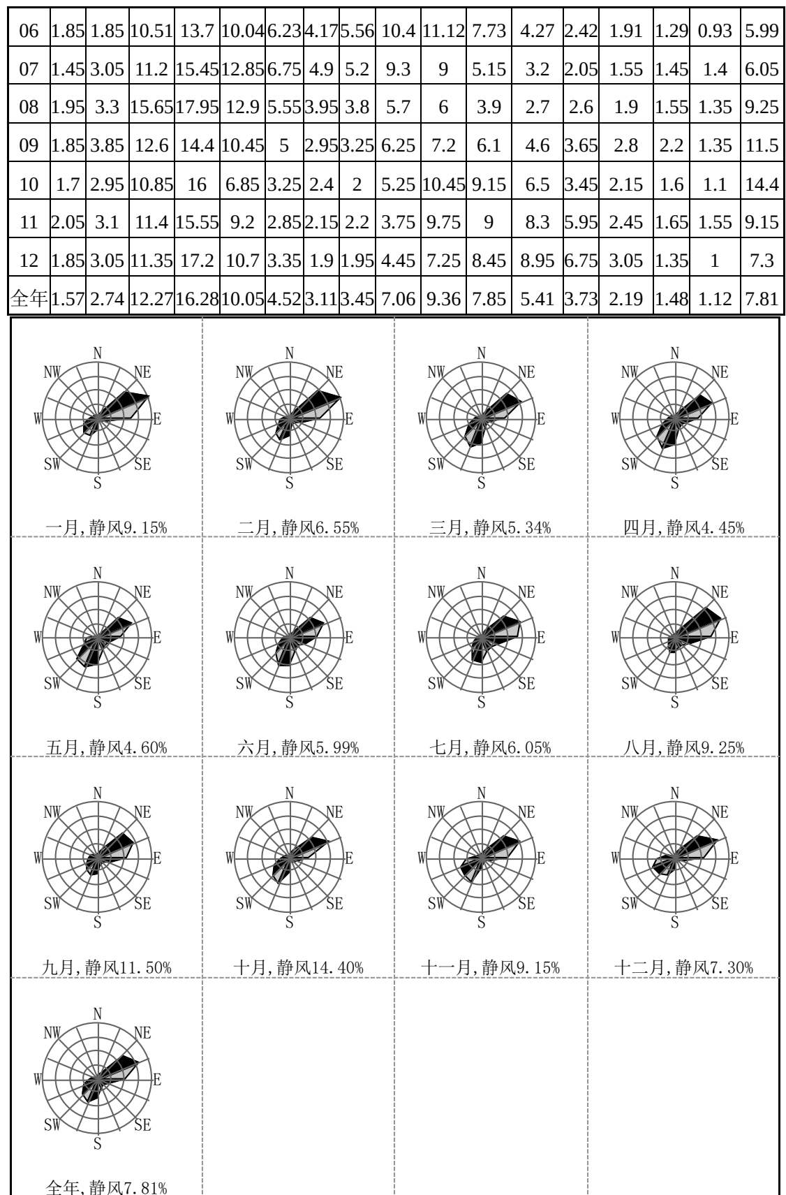
图 5.2-2 新乡风向玫瑰图
