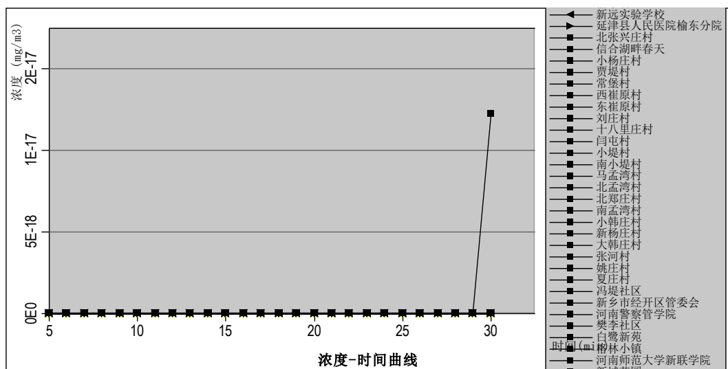
图 6.2-29 最不利气象敏感点氯化氢浓度-时间曲线
