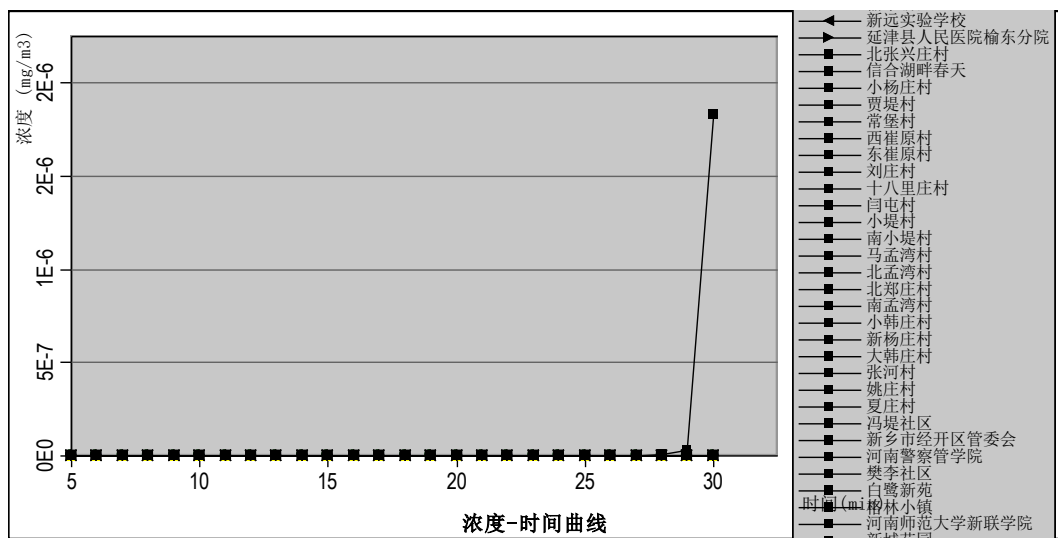
图 6.2-34 最常见气象敏感点甲醇浓度-时间曲线
