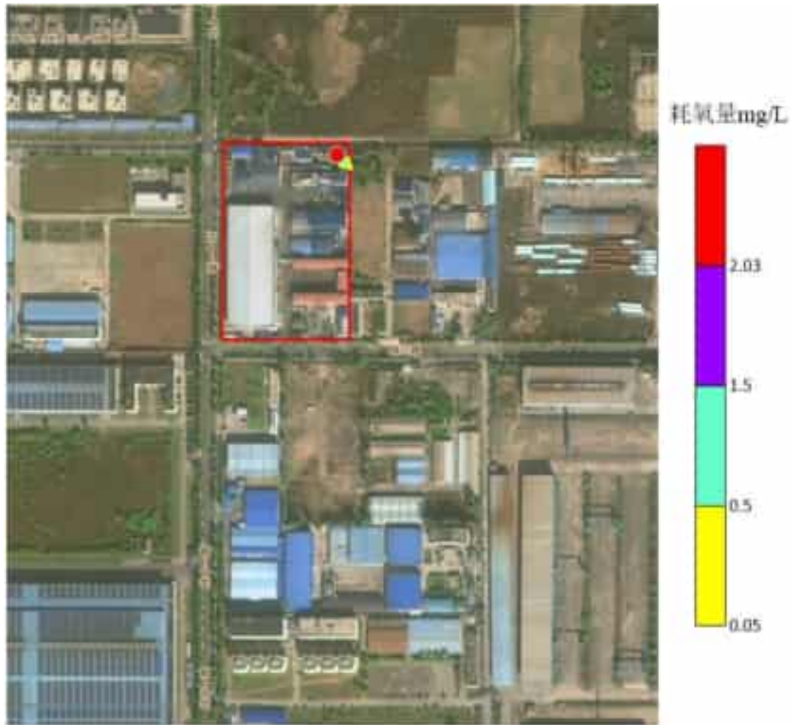
图 5.6-15 100 天污染晕运移分布图
