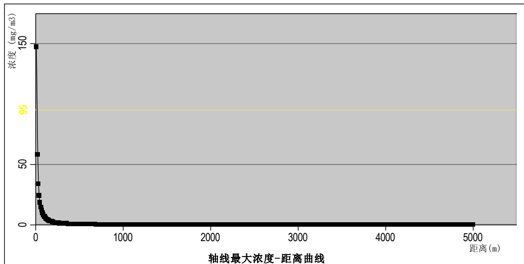
图 6.2-8 最常见气象下风乙腈最大浓度-距离曲线
