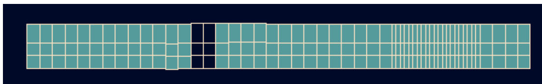
图 5.6-12 模拟区 C-D 剖面垂向剖分图
