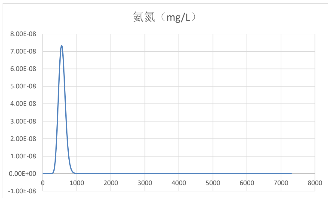
图 5.6-24 厂区下游边界地下水氨氮污染趋势图
