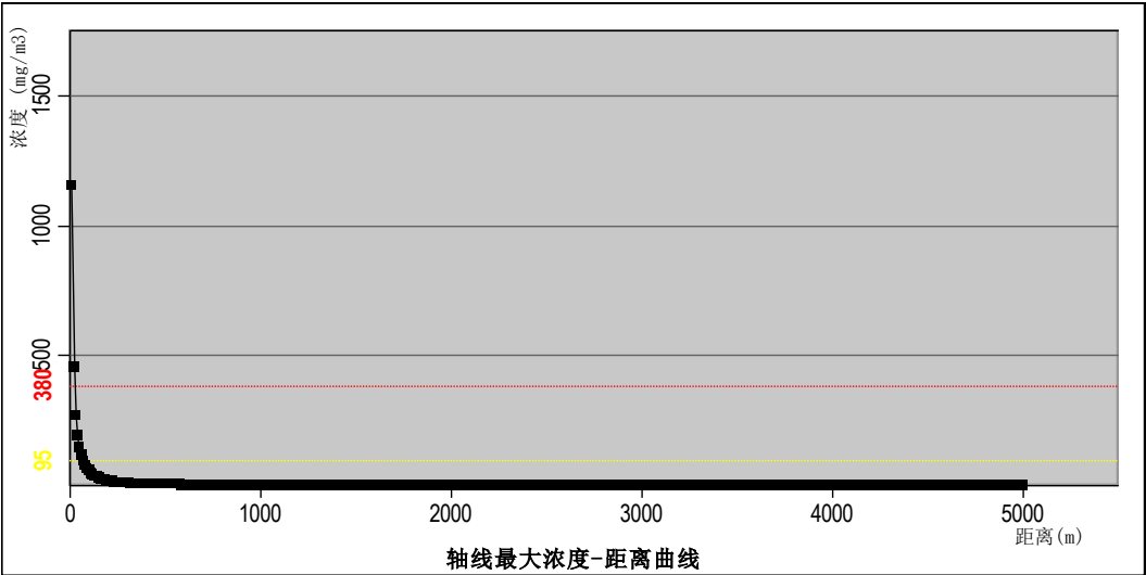
图 6.2-46 最常见气象下风向 CO 最大浓度-距离曲线
