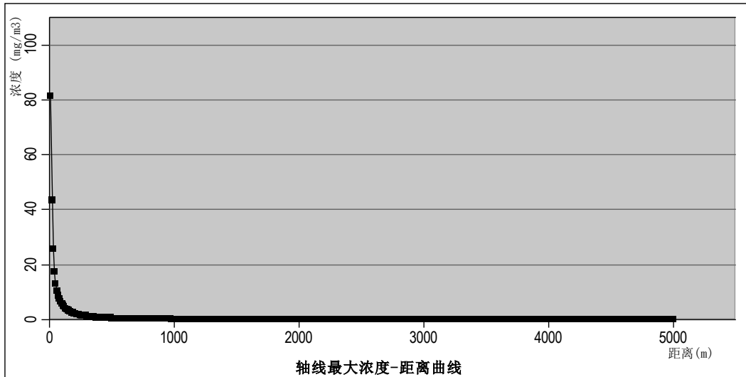
图 6.2-11 最不利气象下风向溴化氢最大浓度-距离曲线
