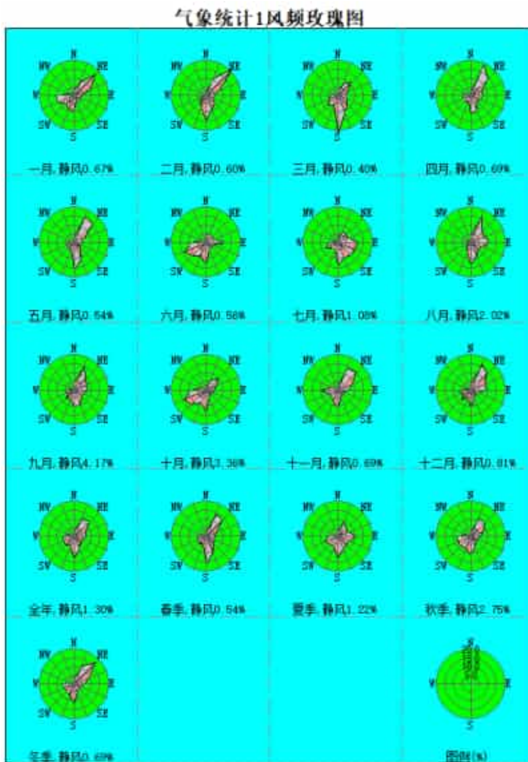
图 5.2-12 全年及各季风向频率图
