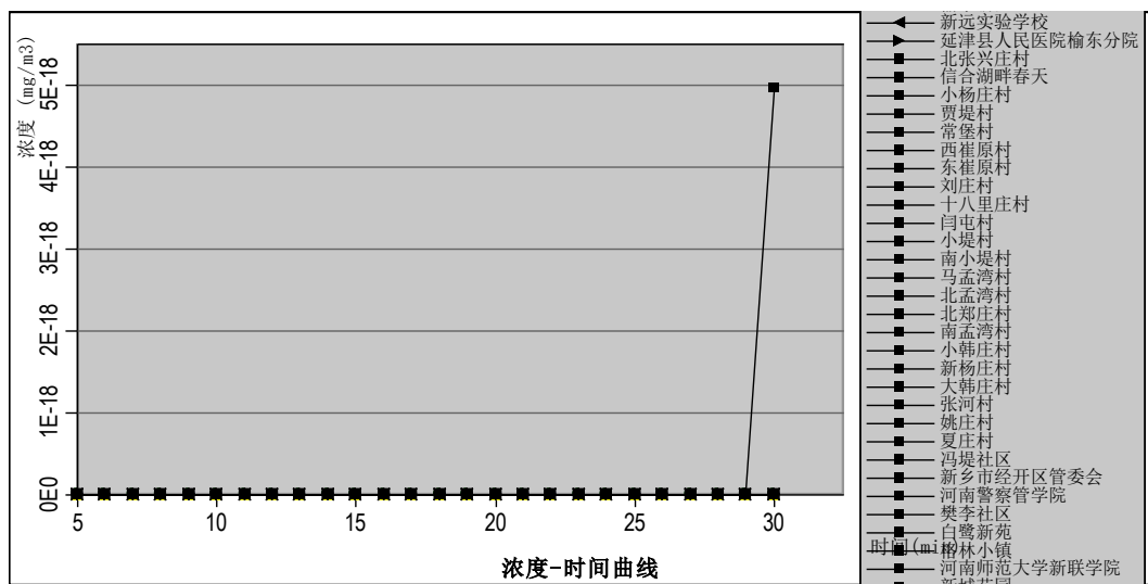
图 6.2-31 最不利气象敏感点甲苯浓度-时间曲线
