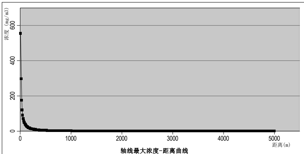
图 6.2-17 最不利气象下风向甲醇最大浓度-距离曲线
