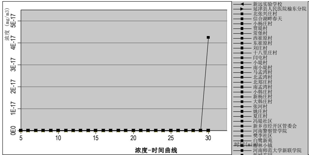
图 6.2-23 最不利气象敏感点乙腈浓度-时间曲线
