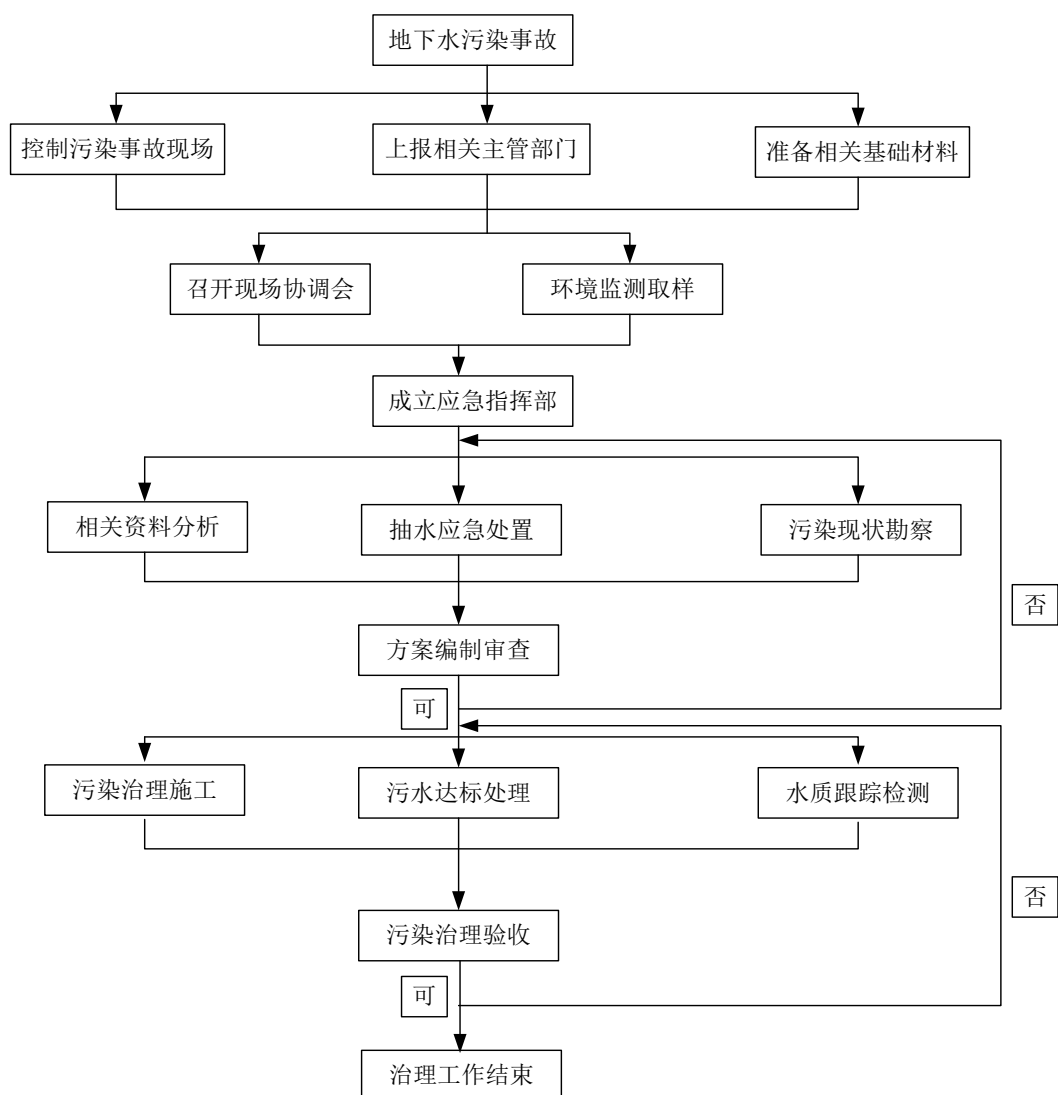
图 6.2-54 地下水污染应急治理程序框图
