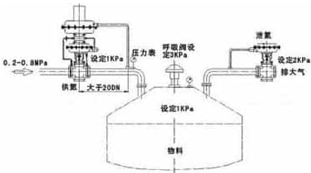
图 3.5-2 罐区氮封装置示意图
