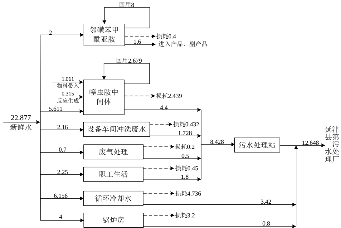
图 3.2-3 现有工程水平衡示意图 单位: \text{m}^3/\text{d}
