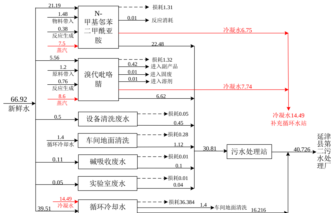
图 3.3-1 本次工程水平衡图 单位: \text{m}^3/\text{d}
