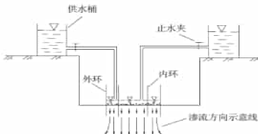
图 5.6-7 双环法渗水试验示意图
