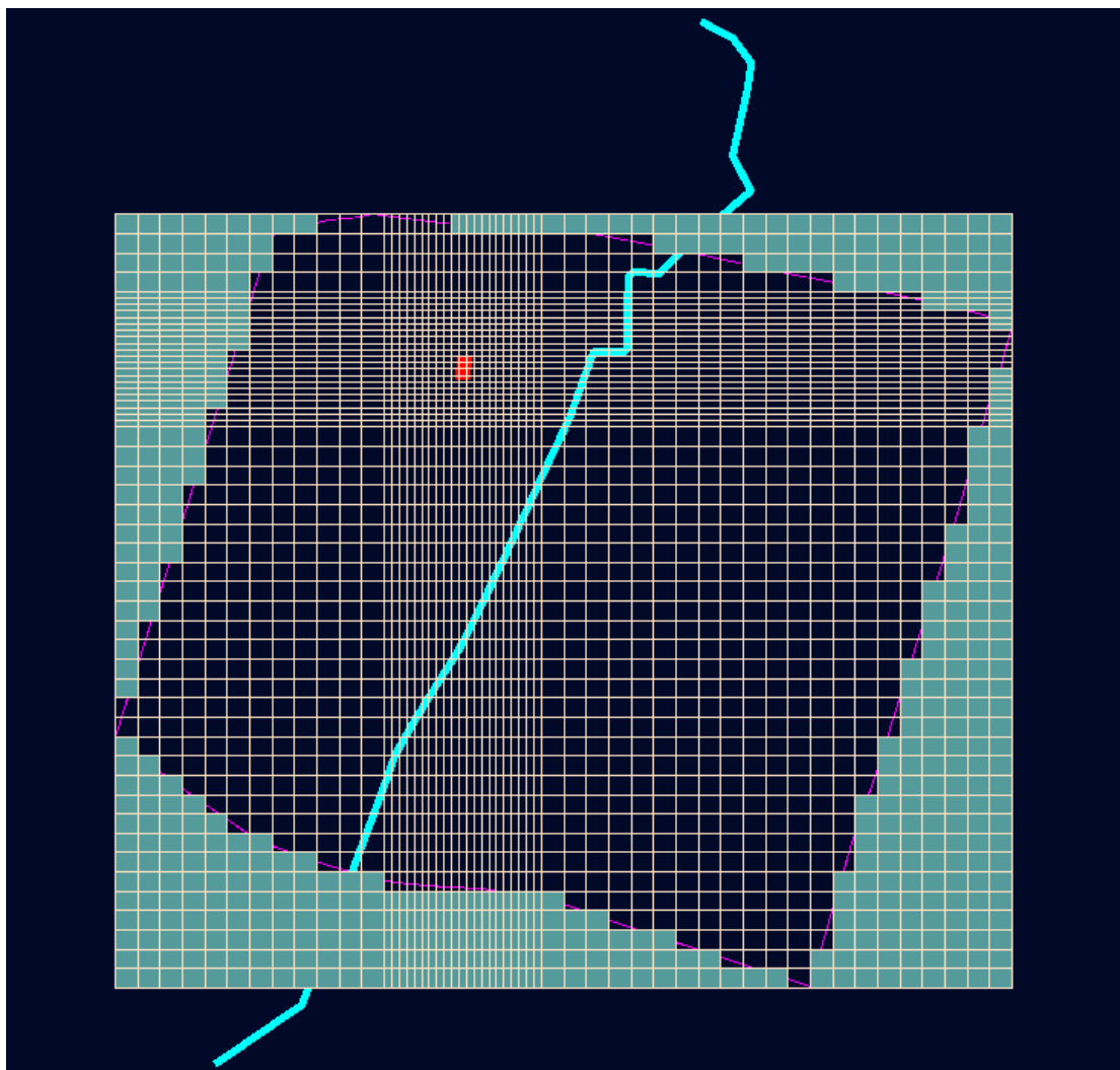
图 5.6-10 模拟计算区范围示意图
