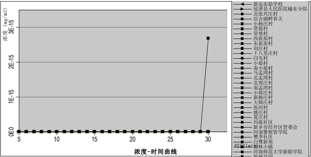
图 6.2-35 最不利气象敏感点一甲胺浓度-时间曲线
