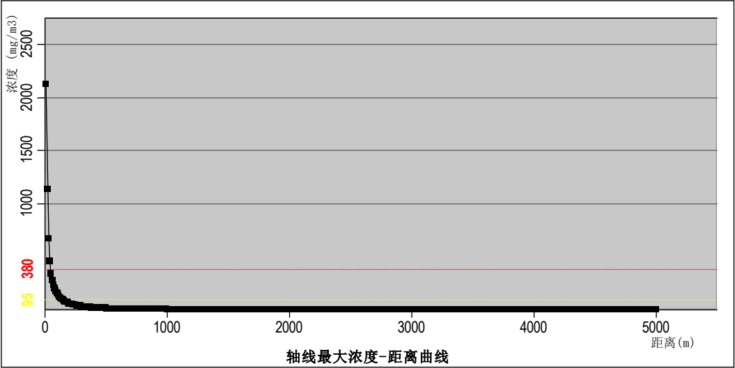
图 6.2-45 最不利气象下风向 CO 最大浓度-距离曲线
