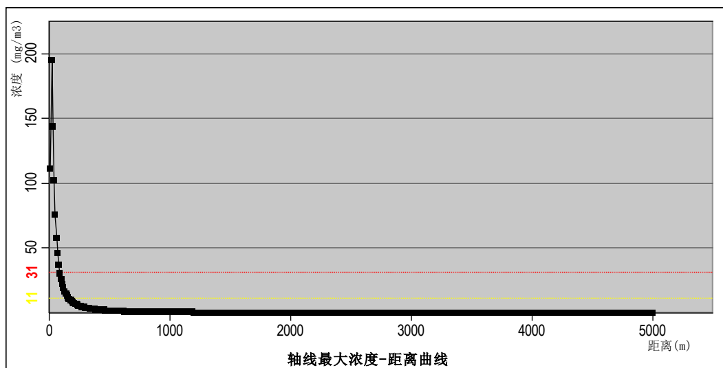
图 6.2-10 最常见气象下风三氯化磷最大浓度-距离曲线
