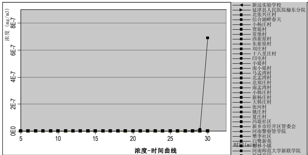
图 6.2-24 最常见气象敏感点乙腈浓度-时间曲线
