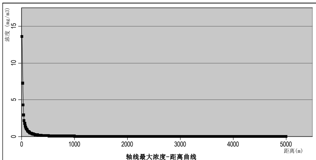
图 6.2-5 最不利气象下风向 DMF 最大浓度-距离曲线
