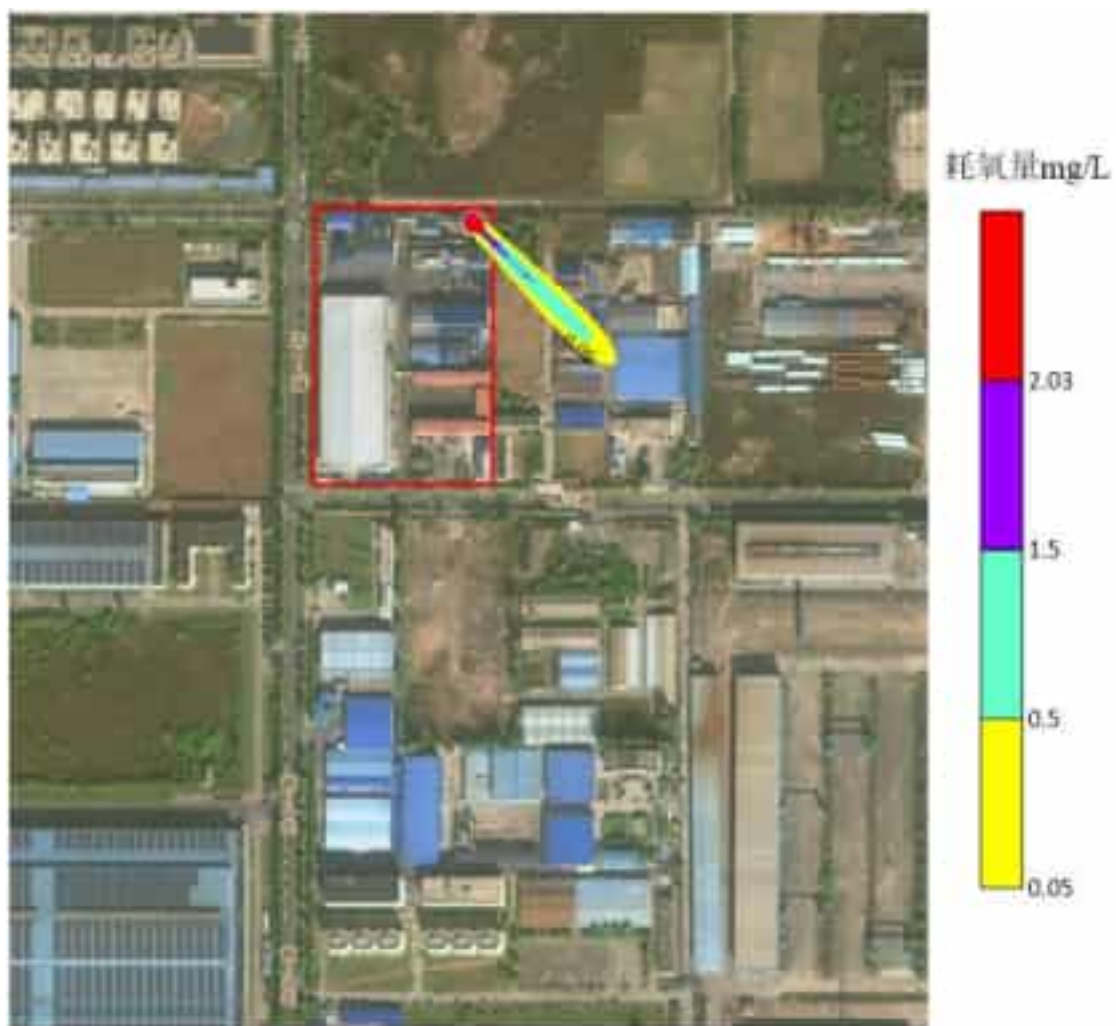
图 5.6-16 1000 天污染晕运移分布图
