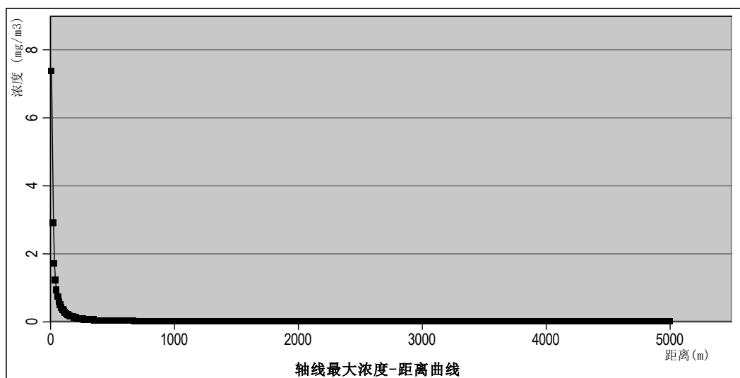
图 6.2-6 最常见气象下风 DMF 最大浓度-距离曲线
