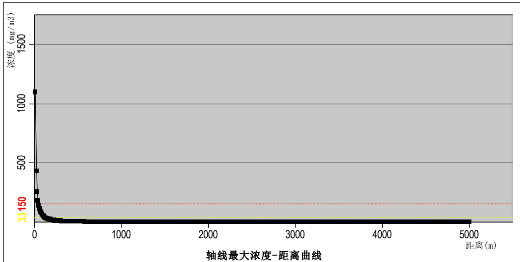
图 6.2-14 最常见气象下风向氯化氢大浓度-距离曲线
