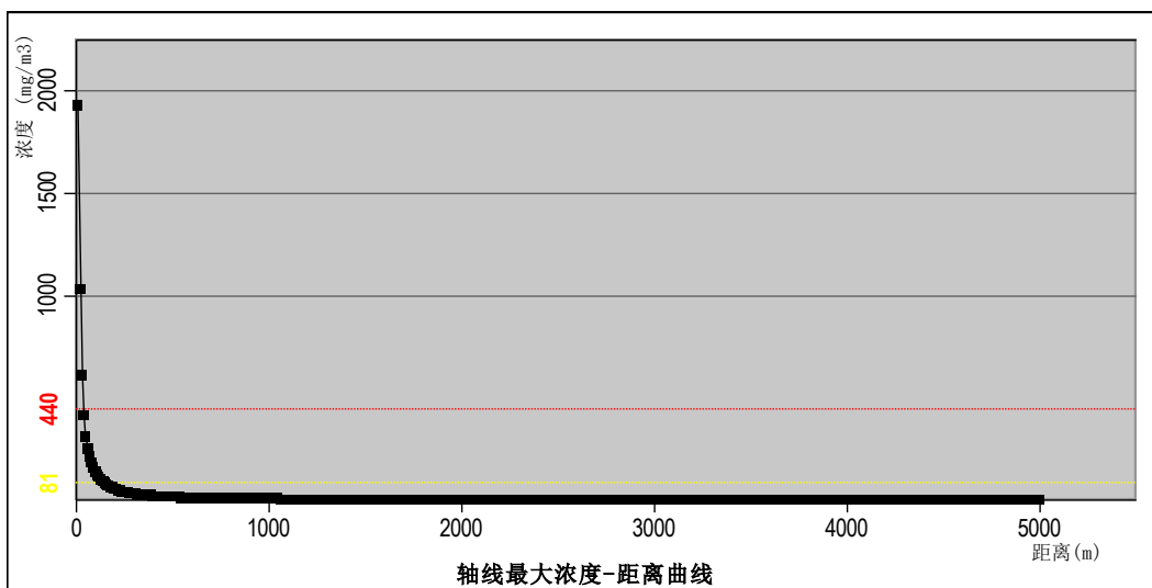
图 6.2-19 最不利气象下风向一甲胺最大浓度-距离曲线
