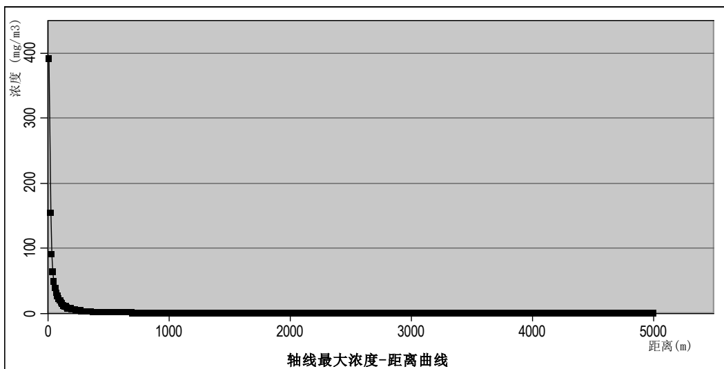
图 6.2-18 最常见气象下风甲醇最大浓度-距离曲线
