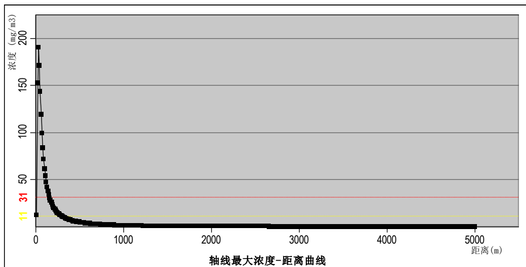
图 6.2-9 最不利气象下风向三氯化磷最大浓度-距离曲线
