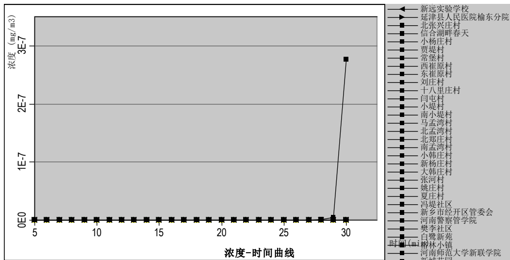
图 6.2-28 最常见气象敏感点溴化氢浓度-时间曲线
