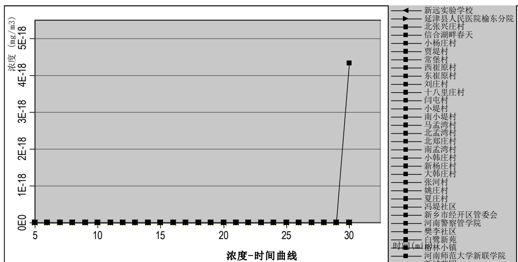
图 6.2-33 最不利气象敏感点甲醇浓度-时间曲线
