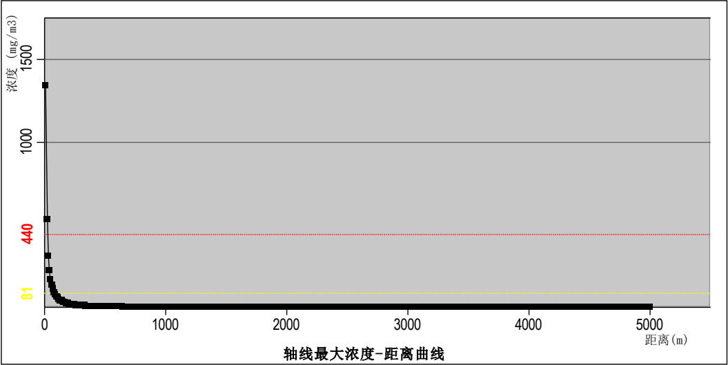
图 6.2-20 最常见气象下风一甲胺最大浓度-距离曲线
