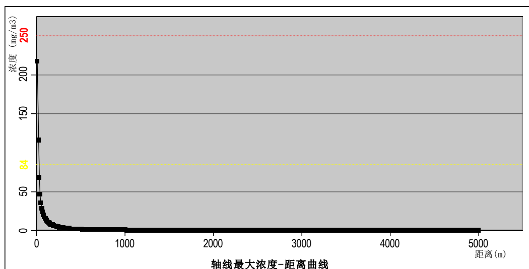
图 6.2-7 最不利气象下风向乙腈最大浓度-距离曲线
