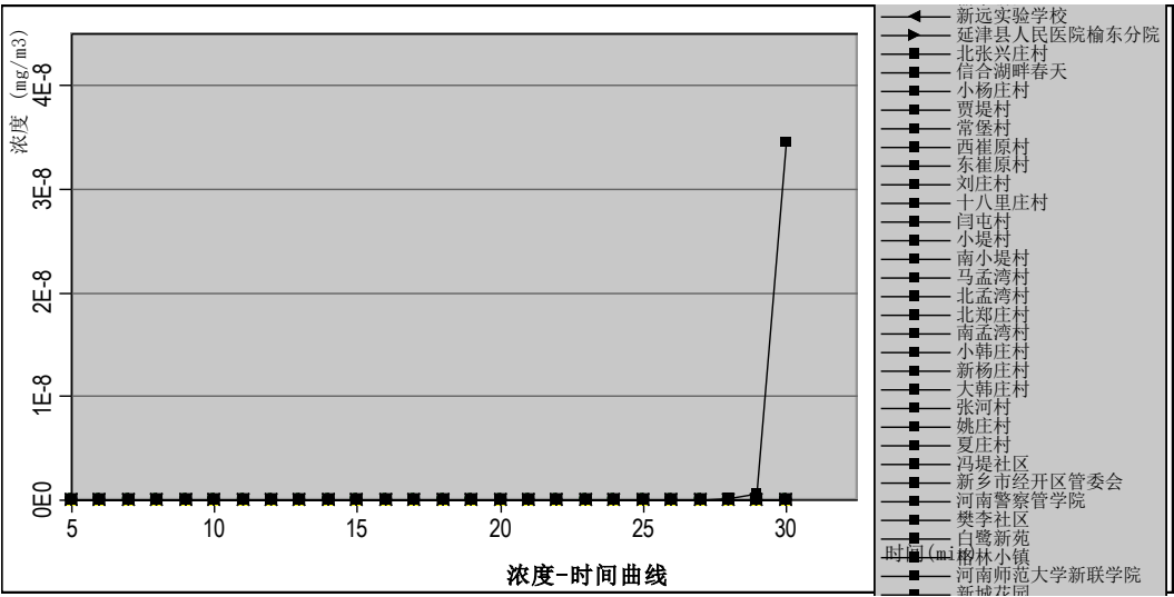
图 6.2-22 最常见气象敏感点 DMF 浓度-时间曲线
