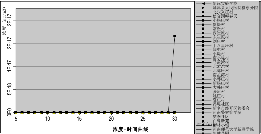
图 6.2-47 最不利气象敏感点 CO 浓度-时间曲线
