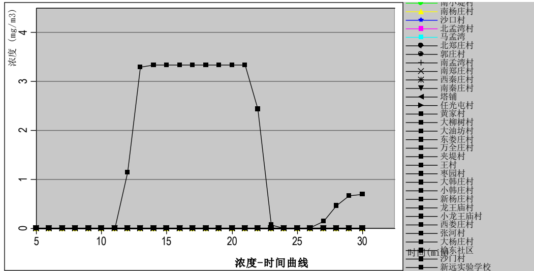
图 6.2-26 最常见气象敏感点三氯化磷浓度-时间曲线
