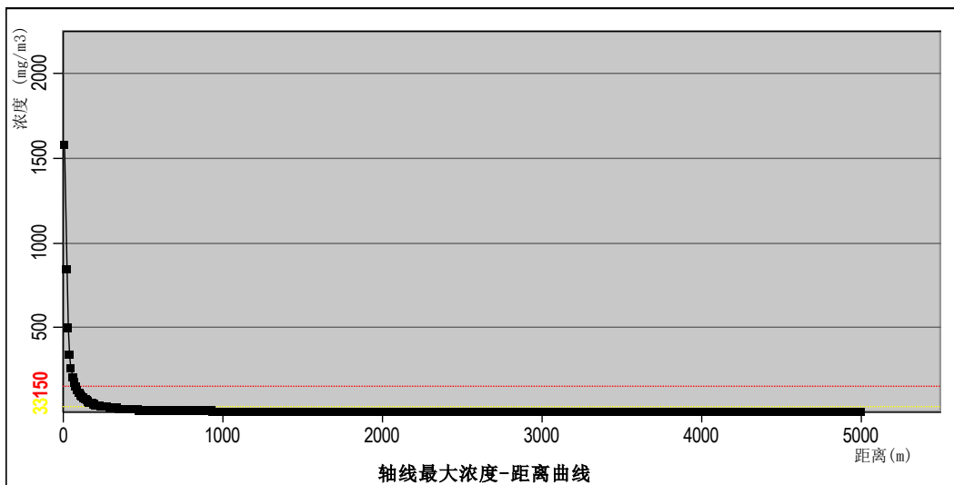
图 6.2-13 最不利气象下风向氯化氢最大浓度-距离曲线
