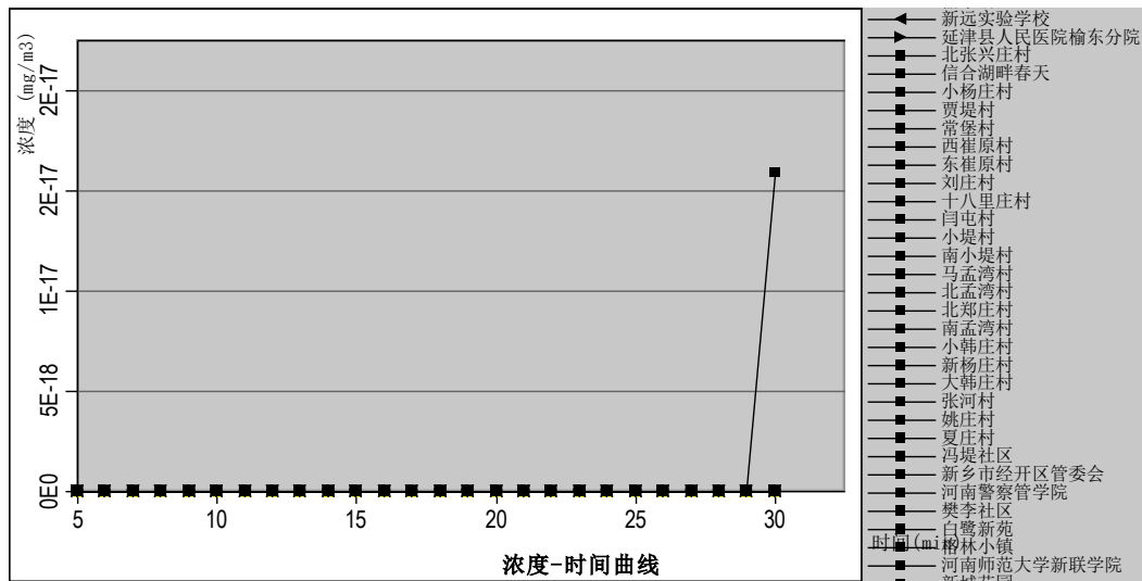
图 6.2-27 最不利气象敏感点溴化氢浓度-时间曲线
