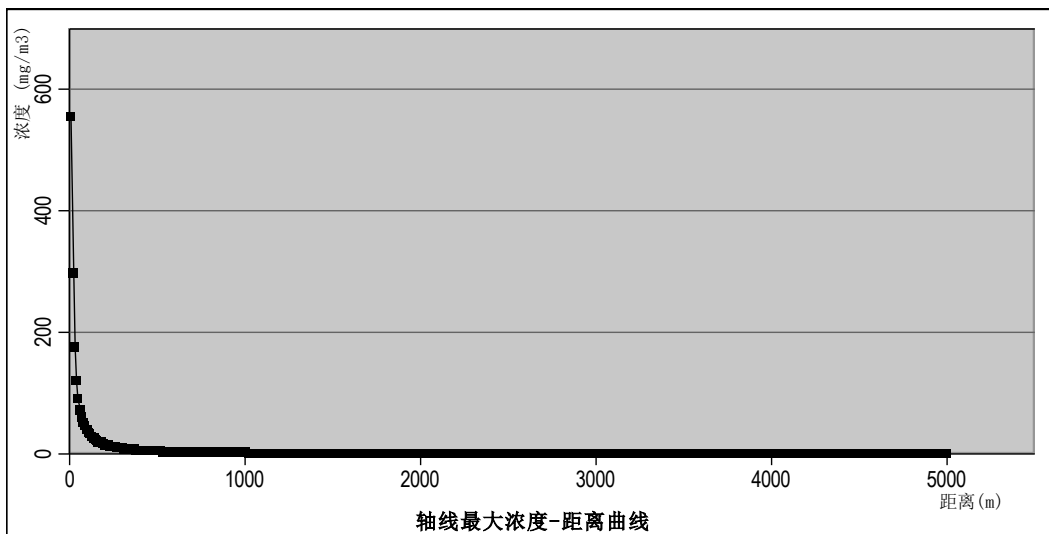
图 6.2-16 最常见气象下风甲苯最大浓度-距离曲线
