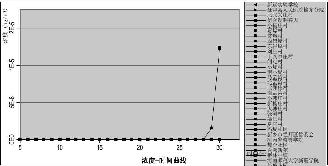
图 6.2-36 最常见气象敏感点一甲胺浓度-时间曲线
