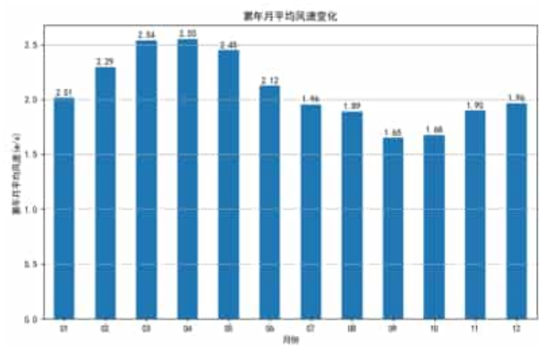
图 5.2-1 新乡月平均风速（单位：m/s）
