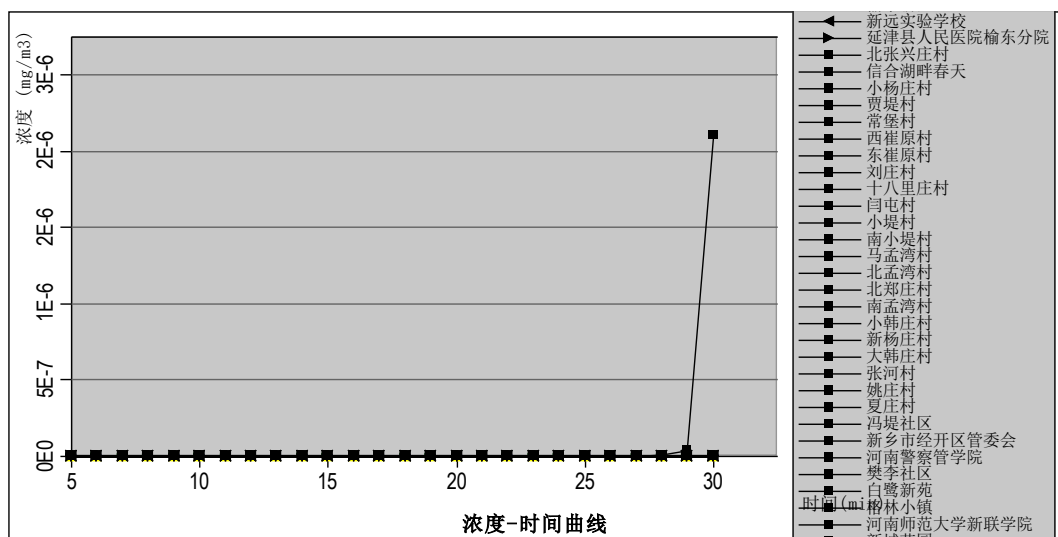
图 6.2-32 最常见气象敏感点甲苯浓度-时间曲线
