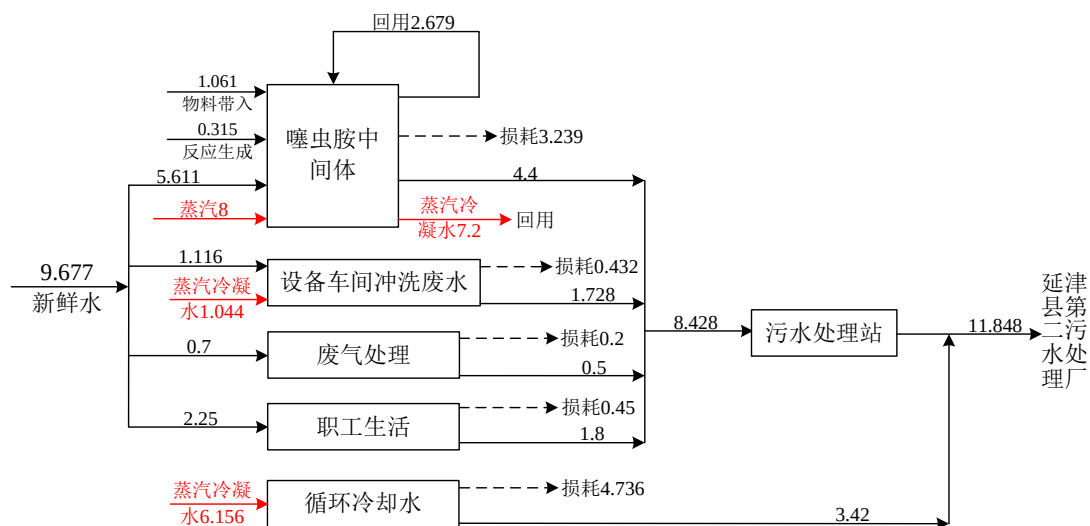
图 3.2-6 “以新带老”后现有工程水平衡示意图
