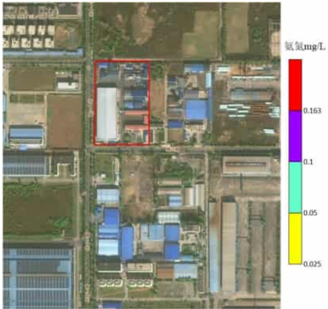
图 5.6-20 1000 天污染晕运移分布图
