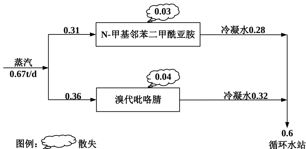
图 3.3-3 本次工程蒸汽/凝水平衡图 单位：t/h
