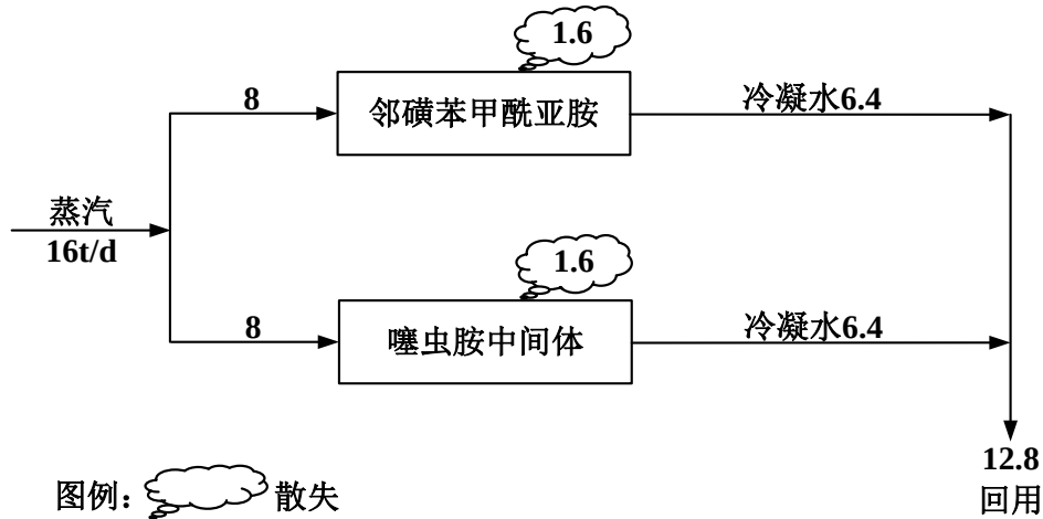
图 3.2-4 现有工程蒸汽平衡示意图 单位: \text{t}/\text{d}
