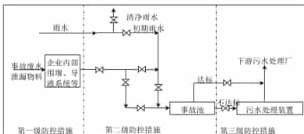
图 6.2-53 三级防控系统设置示意图
